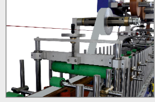
ÇİFT YÜZEY KORUYUCU BANT KAPLAMA İSTASYONU DOUBLE SURFACE PROTECTIVE TAPE LAMINATION STATION ДВУХСТОРОННЯЯ СИСТЕМА РАЗМОТКИ И НАНЕСЕНИЯ ЗАЩИТНОЙ ПЛЕНКИ
